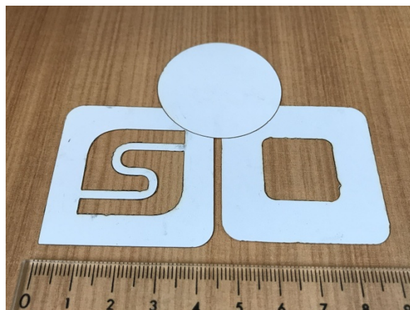
2 - Silný bílý papír 0,15 mm, F 10 mm/s, Pwr 255
