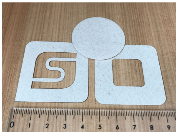
3 - Hnědý papír 0,1 mm, F 15 mm/s, Pwr 255
