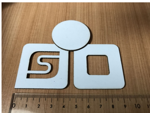
5 - karton Solid (bílá strana) 1,1 mm, F 15 mm/s, Pwr 255
