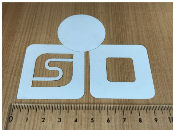
1 - Bílý papír 0,1 mm, F 18 mm/s, Pwr 255
