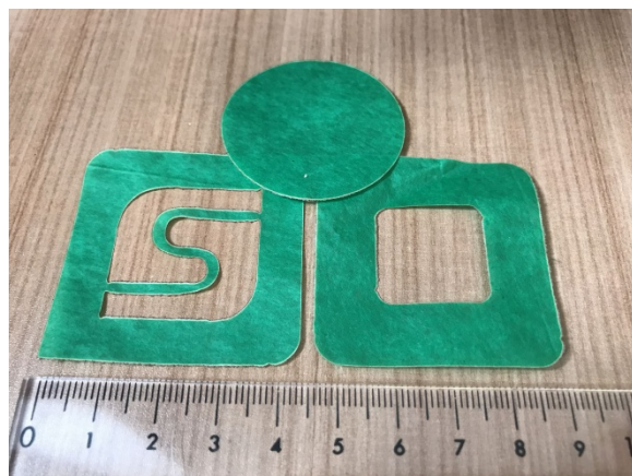
4 - Čínský papír 0,05 mm, F 30 mm/s, Pwr 255
