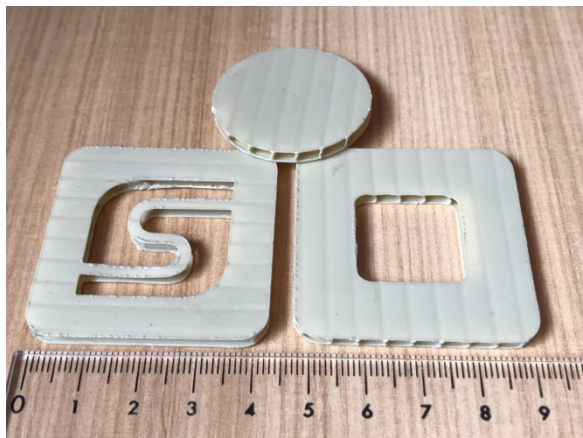
19 - Coroplast světle hnědá 3,5 mm, F 3 mm/s, Pwr 255
